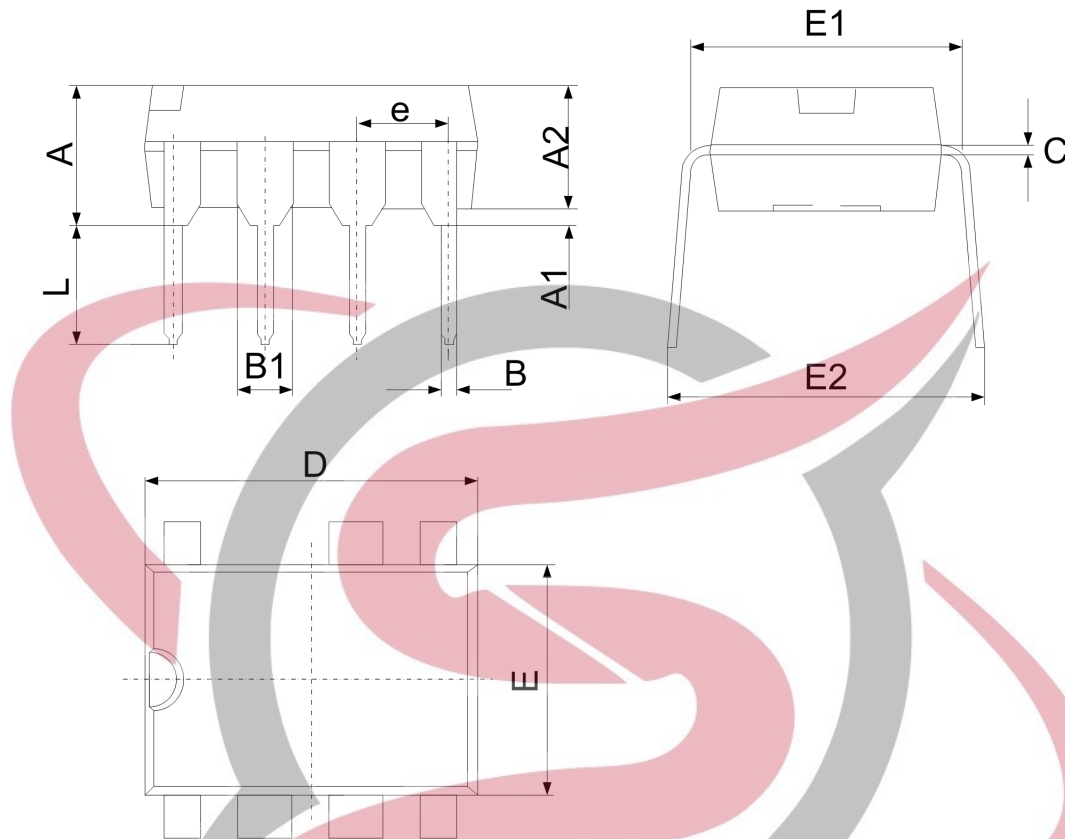
DIP-7
